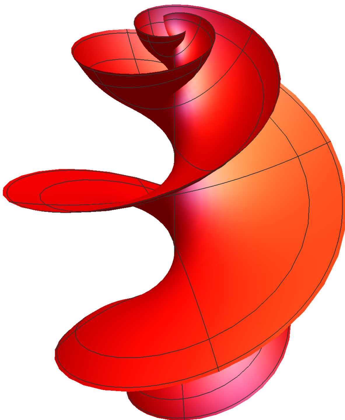
Figura 3.6: Elicoide iperbolico
