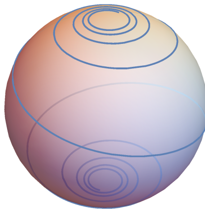
Figura 3.2: Una spirale sferica
