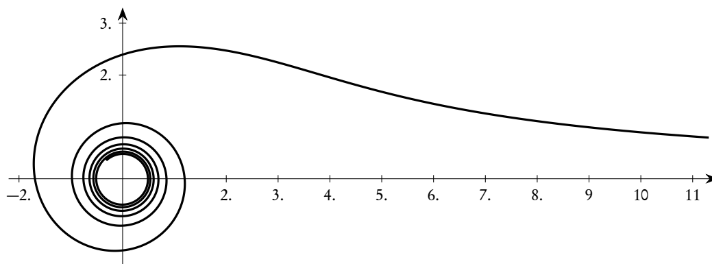
Figura 2.12: Il lituus
