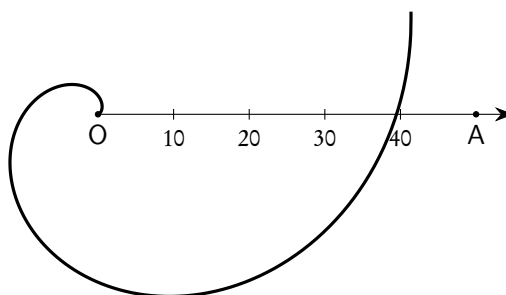
Figura 1.7: La curva r = \vartheta^2 in coordinate polari
