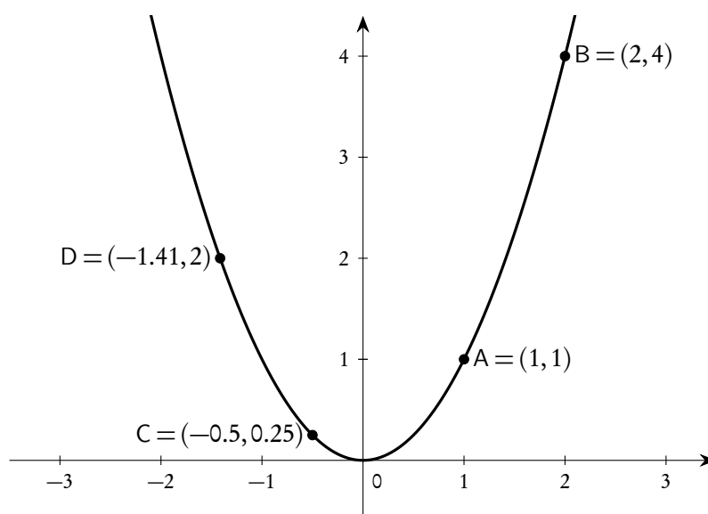
Figura 1.4: Grafico di y = x^2
