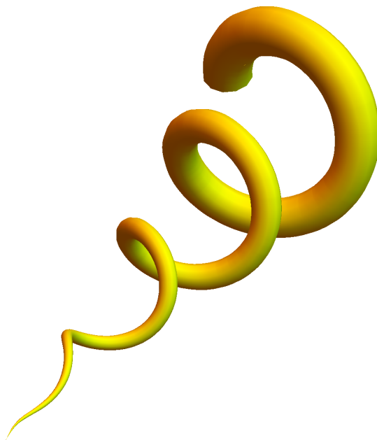
Figura 3.4: Figura costruita a partire da un'elica conica
