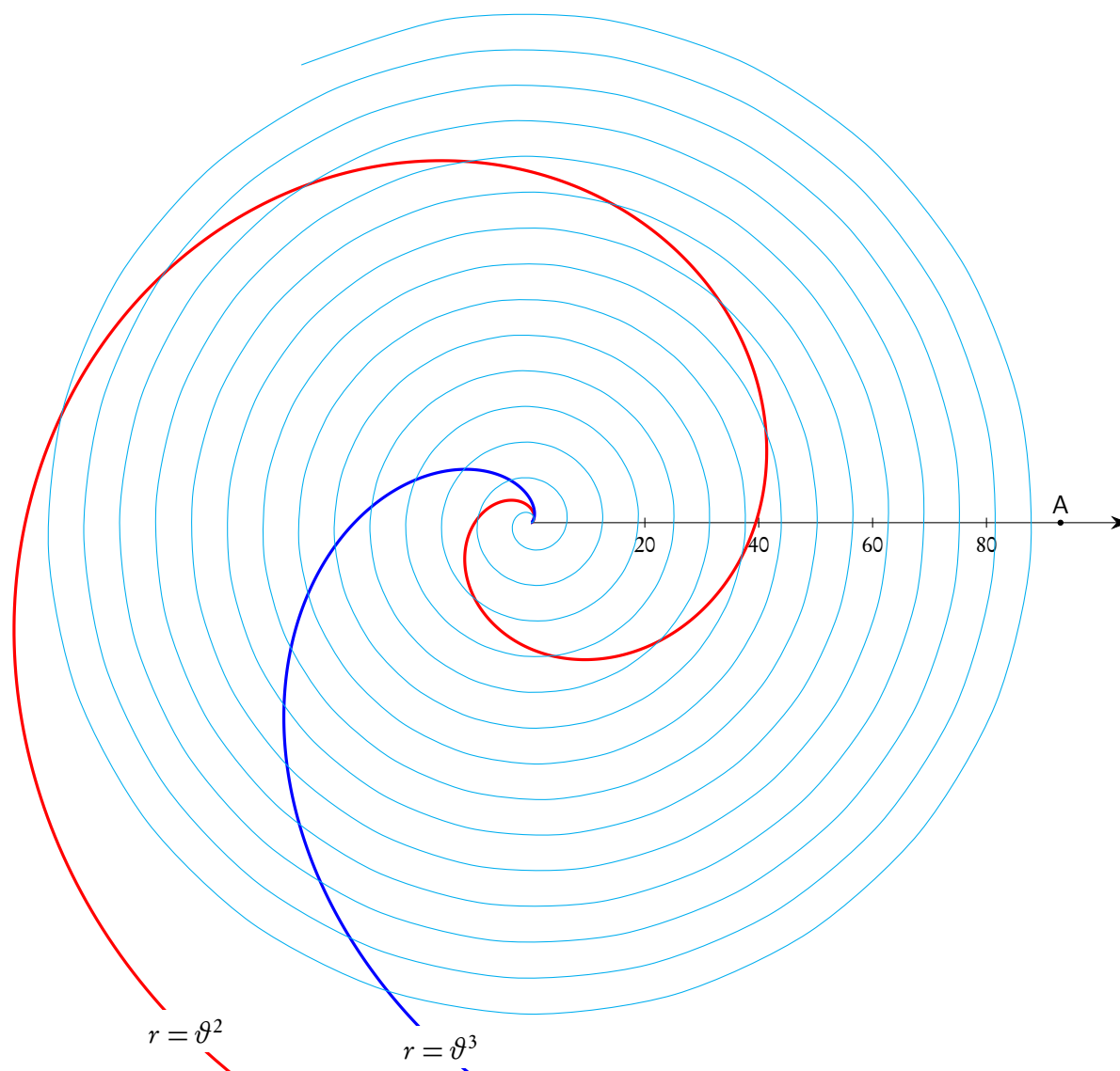
Figura 2.2: Spirali del tipo r = \vartheta^n
