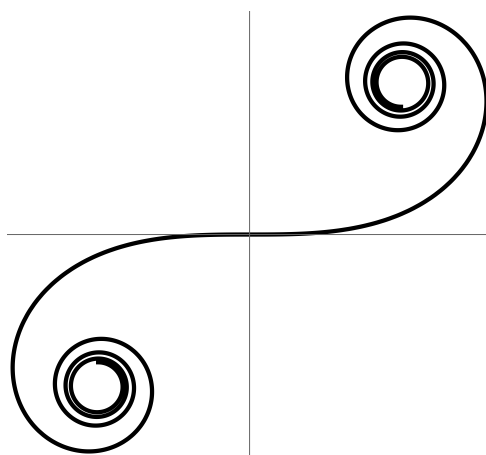
Figura 2.13: Una spirale di Cornu
