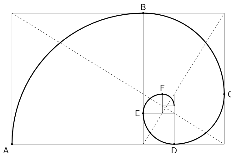
Figura 2.9: Pseudospirale aurea e rettangolo aureo
