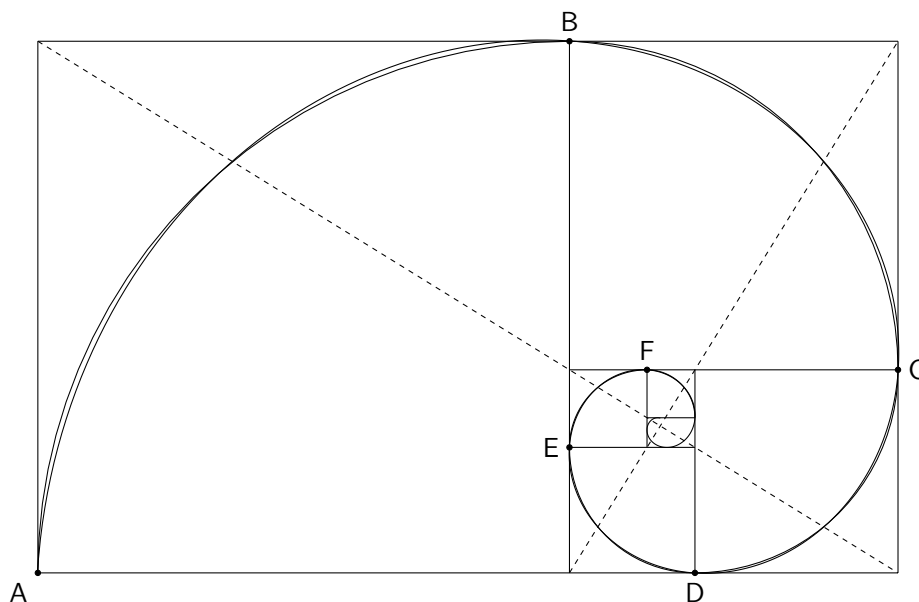
Figura 2.10: Confronto tra spirale e pseudospirale aurea nel rettangolo aureo
