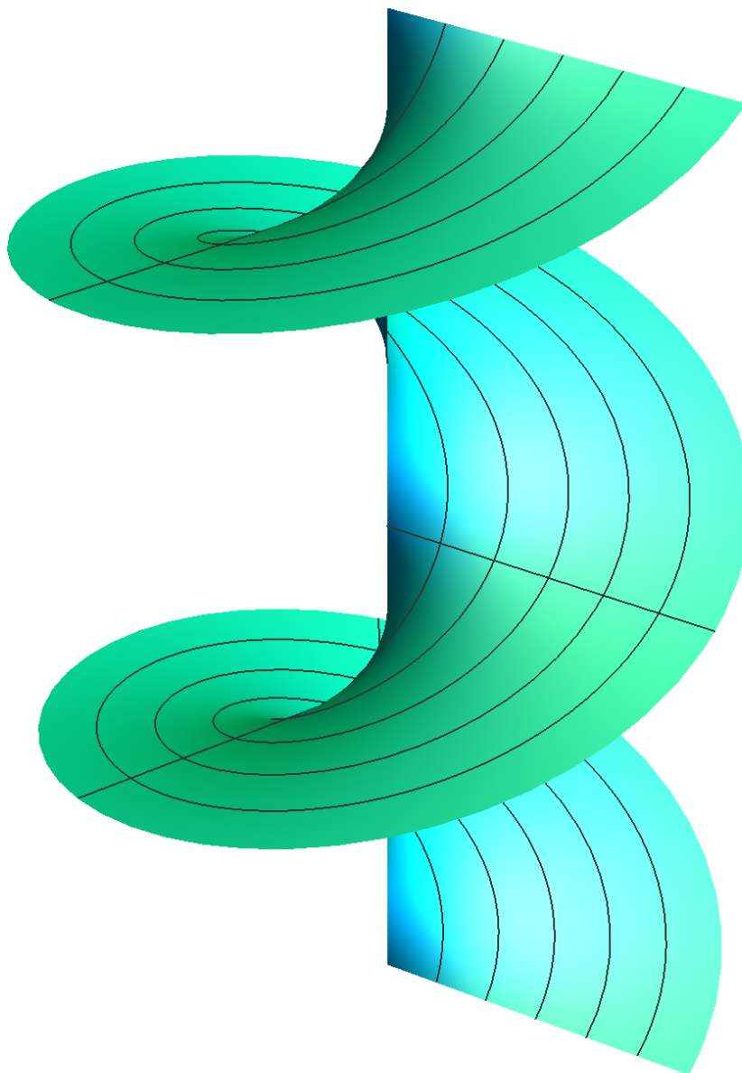
Figura 3.5: Elicoide circolare
