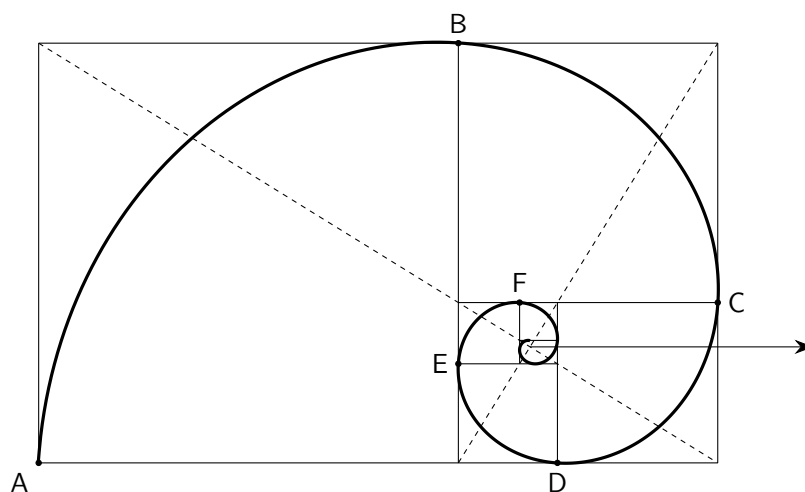
Figura 2.8: Spirale aurea e rettangolo aureo
