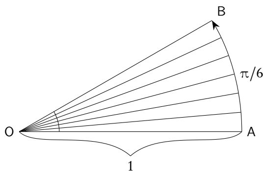
Figura 1.2: Angolo di 30^\circ e lunghezza dell'arco descritto dal lato \overline{OA}
