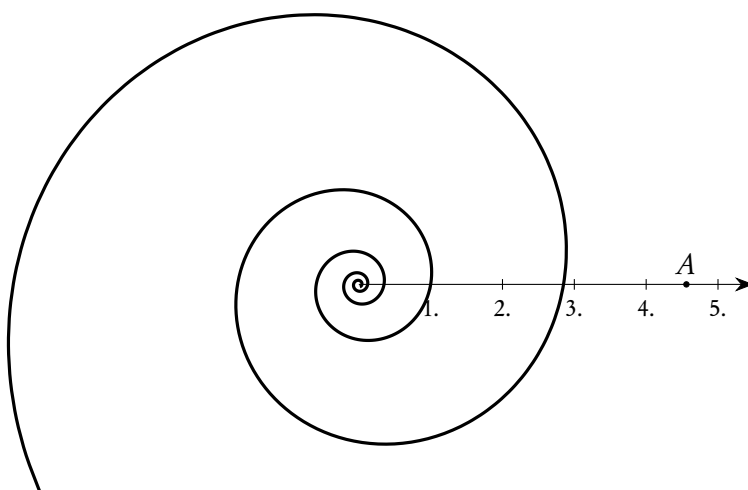
Figura 2.6: Spirale logaritmica r = e^{\vartheta/6}
