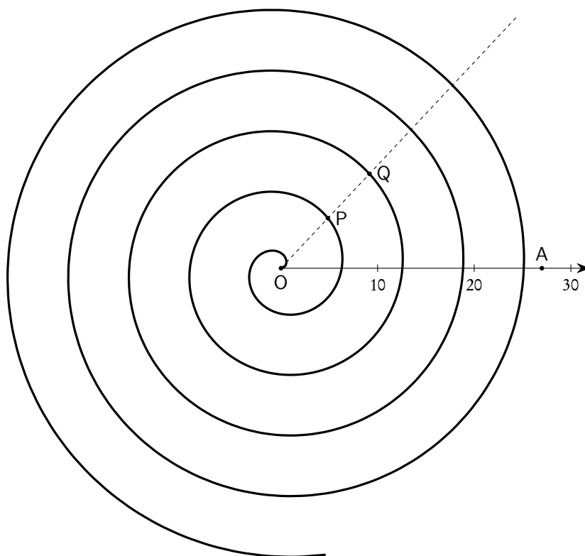
Figura 2.1: La spirale di Archimede
