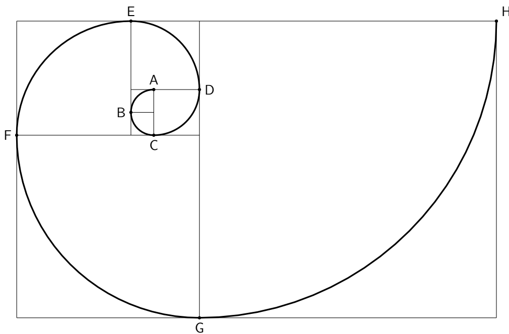
Figura 2.11: La spirale di Fibonacci
