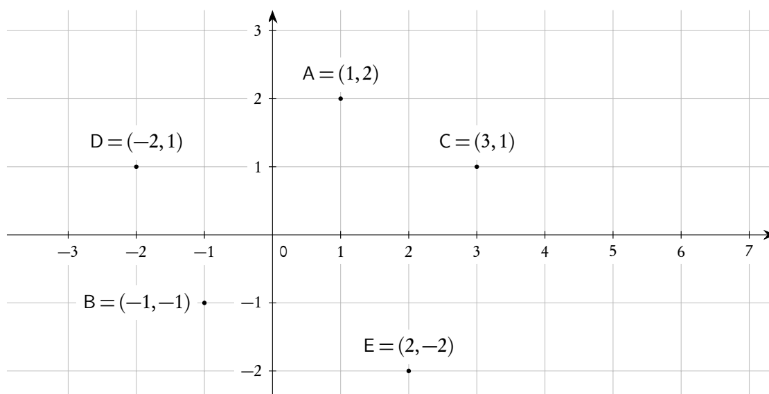
Figura 1.3: Punti e loro coordinate cartesiane nel piano
