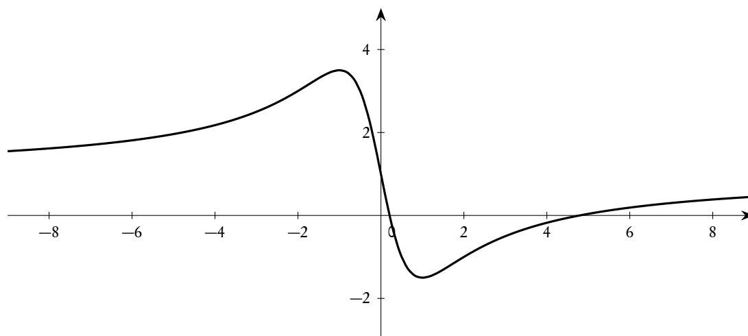
Figura 1.5: Grafico di y = (x^2 - 5x + 1)/(x^2 + 1)
