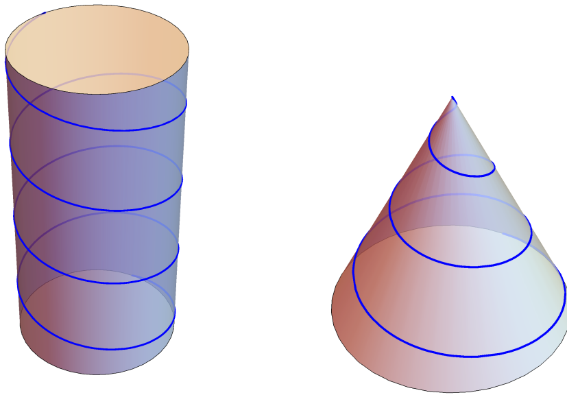
Figura 3.1: Un'elica cilindrica e un'elica conica
