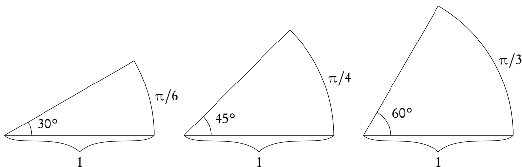
Figura 1.1: Angoli e loro misura in radianti
