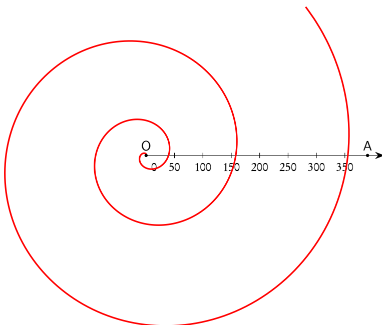
Figura 2.3: La spirale r = \theta^2 , con un maggiore numero di spire
