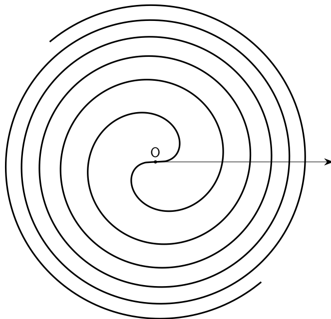
Figura 2.14: La spirale di Fermat
