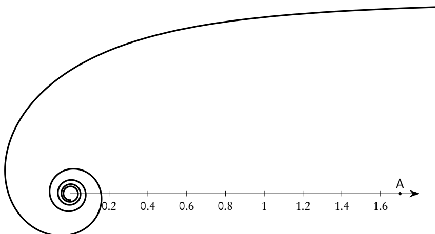
Figura 2.5: La spirale iperbolica
