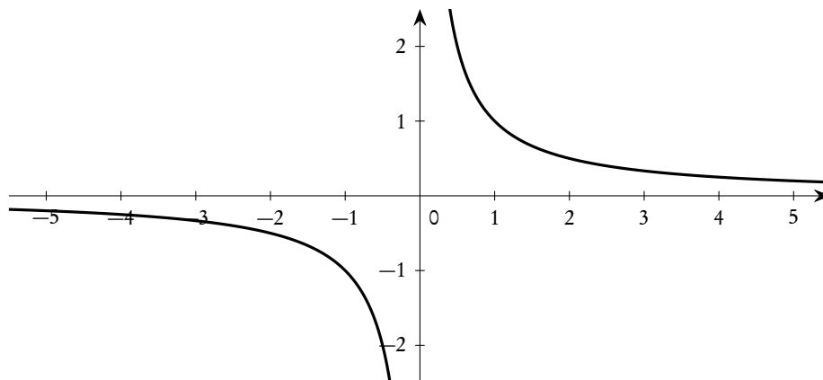
Figura 2.4: Proporzionalità inversa in coordinate cartesiane
