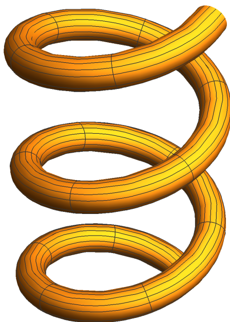
Figura 3.3: Figura costruita a partire da un'elica cilindrica
