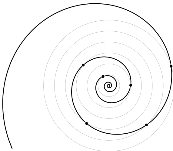
Figura 2.7: Proprietà delle spirali logaritmiche
