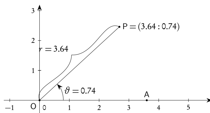
Figura 1.6: Coordinate polari
